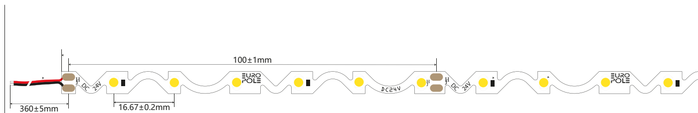
schéma en coupe de la bande
